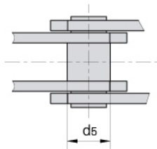
without rollers. ohne Rollen
