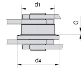
with F flanged rollers type mit F-Bundlaufrollen
